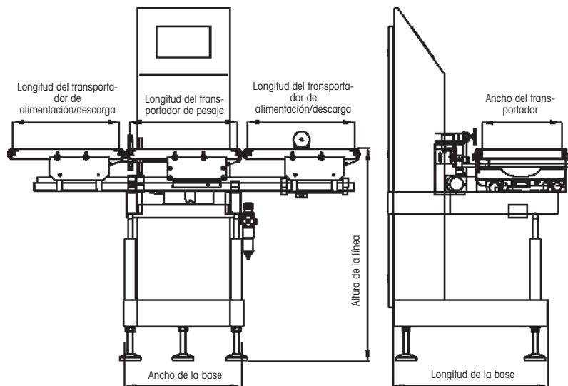
Esquema típico de la XC3
